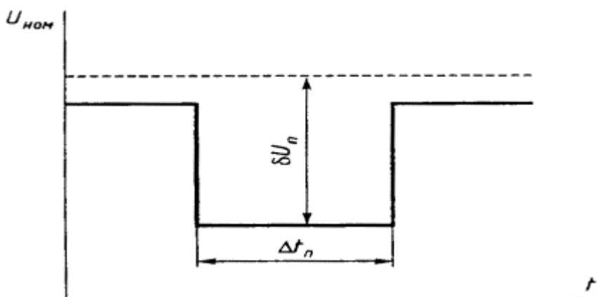
Рисунок Б.2 - Провал напряжения
