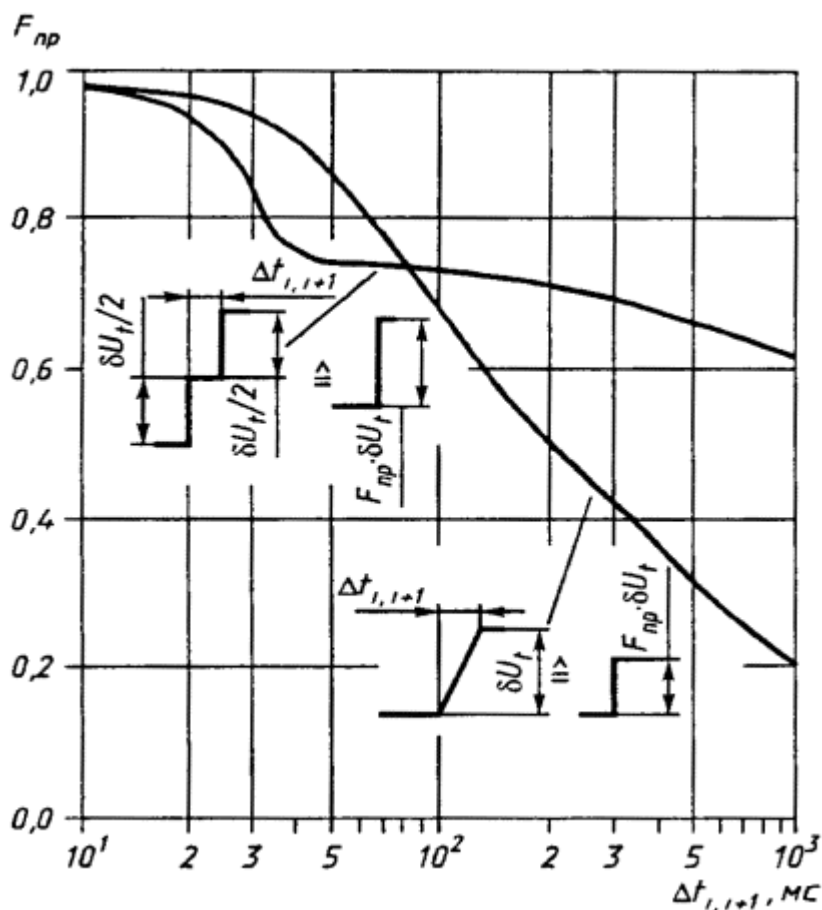
Рисунок В.1 - Коэффициент приведения F_{пр} для периодических колебаний напряжения, имеющих двухступенчатую и пилообразную форму
