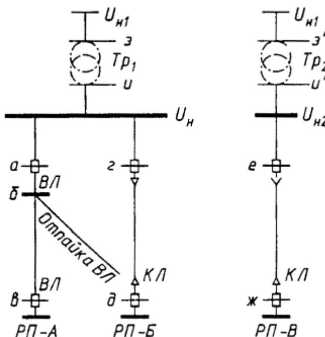
Рисунок Д.1 - Точки присоединения электрической сети общего назначения
