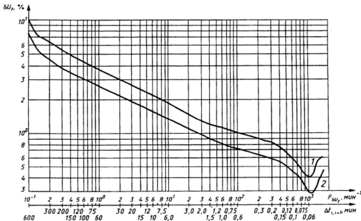
Рисунок 1 - Предельно допускаемые размахи изменений напряжения в зависимости от частоты повторения изменений напряжения за минуту для колебаний напряжения, имеющих форму меандра
