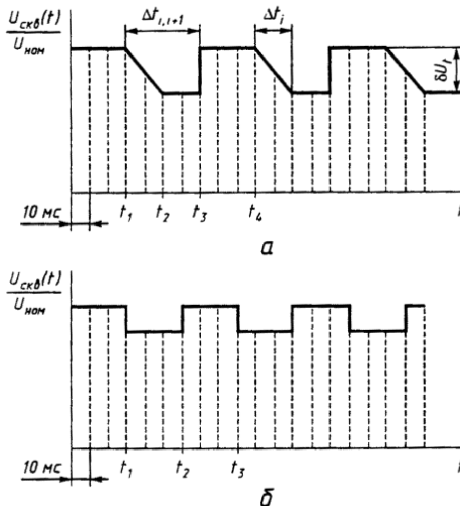
Рис. Б.1 - Колебания напряжения произвольной формы (а) и имеющие форму меандра (б)
