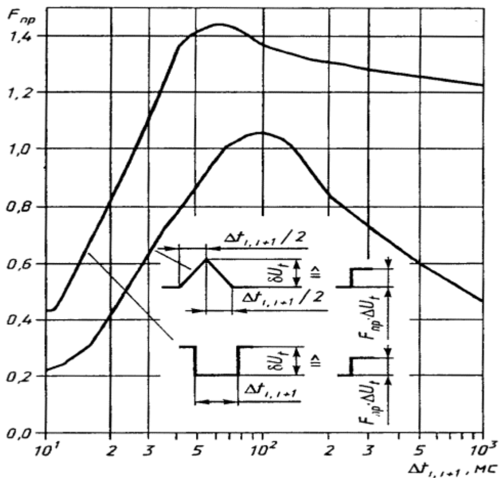
Рисунок В.2 - Коэффициент приведения F_{пр} для прямоугольных и треугольных периодических колебаний напряжения
