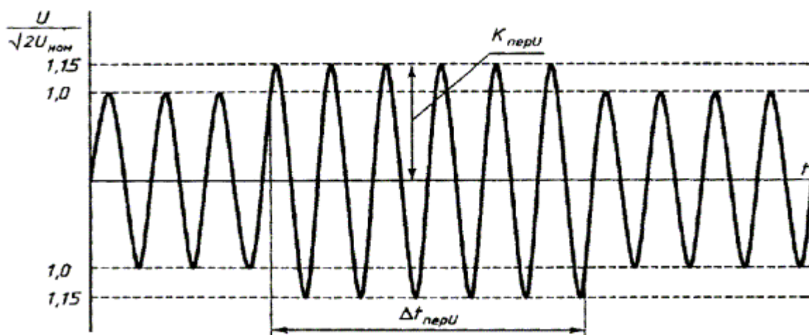
Рисунок Б.4 - Временное перенапряжение
