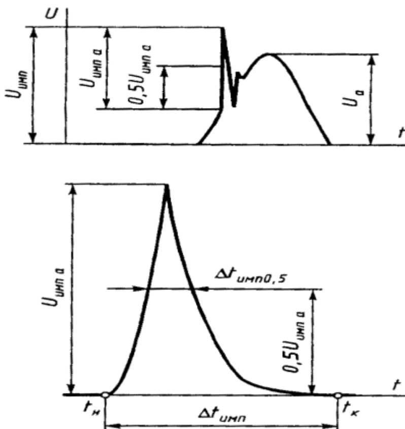
Рисунок Б.3 - Параметры импульсного напряжения
